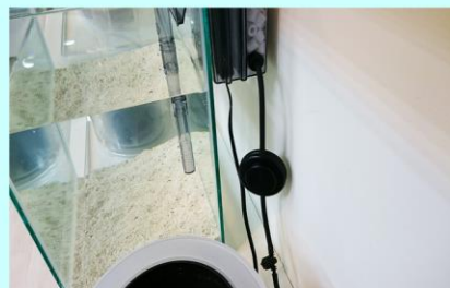
過濾盤及小開關閥接續
